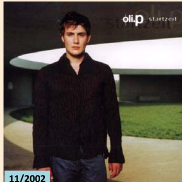
Startzeit
